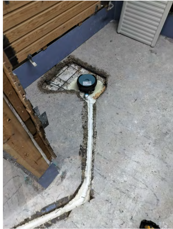
22 - Sauna. Kuivakaivo ja yhdysputki asennettu suunnitelman mukaisesti - Petteri Hujanen - 15.04.2026
