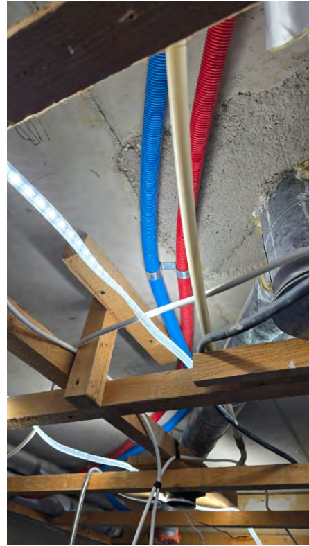
20 - Kuva 1: PEX-käyttövesiputkien asennus ja kannakointi (tarkastettu – ok) - Petteri Hujanen - 16.04.2026
