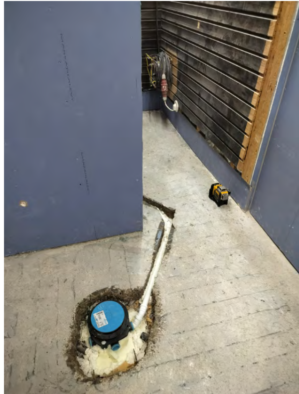
24 - Kph. Lattiakaivo ja yhdysputki kuivakaivolle asennettu suunnitelman mukaisesti - Petteri Hujanen - 15.04.2026
